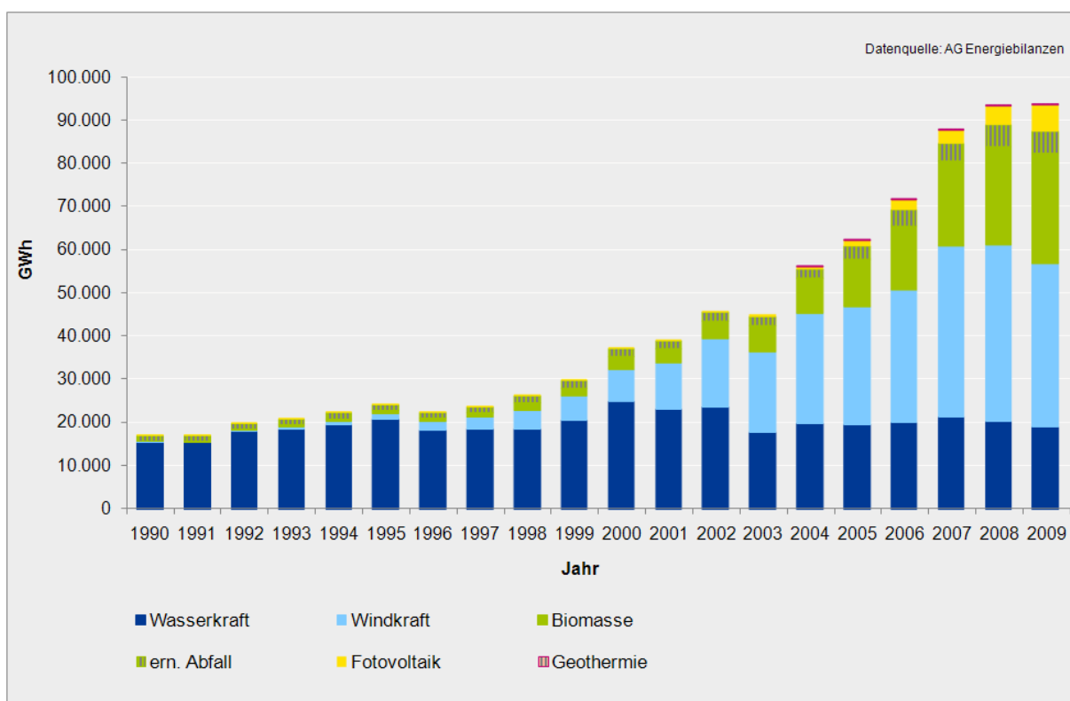
Abbildung A 2.2.4-3: Stromerzeugung auf Basis erneuerbarer Energien nach Energieträgern 1990 bis 2009, in GWh
