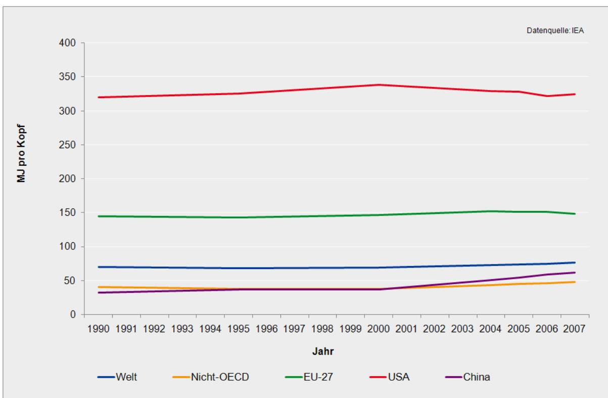
Abbildung A 2.1.1-2: Pro-Kopf Primärenergieverbrauch nach Regionen 1990 bis 2007, in MJ pro Kopf
