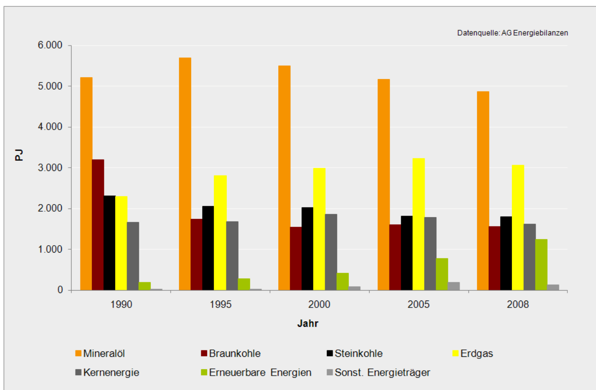
Abbildung A 2.2.2-1: Primärenergieverbrauch nach Energieträgern 1990, 1995, 2000, 2005 und 2008, in PJ
