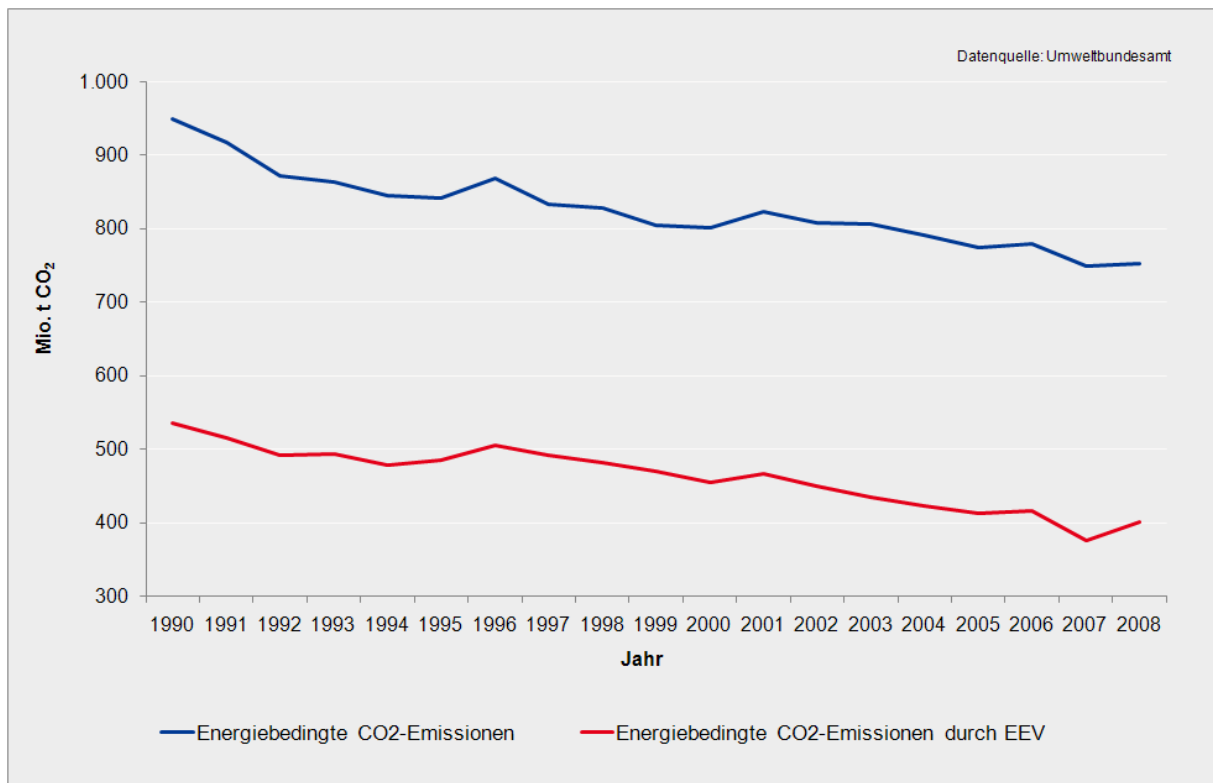
Abbildung A 2.2.3-1: Energiebedingte CO 2 -Emissionen 1990 bis 2008, in Mio t CO 2
