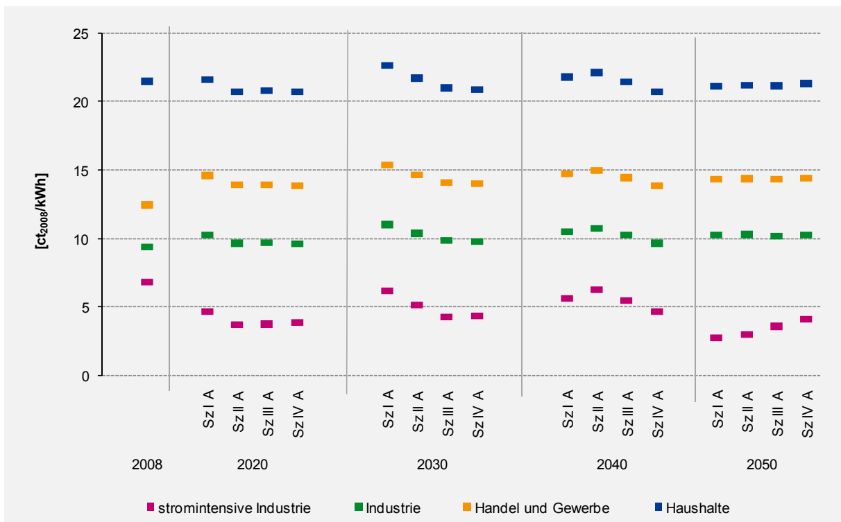
Abbildung 3.2.3.3-3: Endverbraucherpreise in den Szenarien im Zeitverlauf, 2008-2050, in ct 2008 /kWh (2008 historischer Wert gemäß EUROSTAT, EEX und Amprion)
