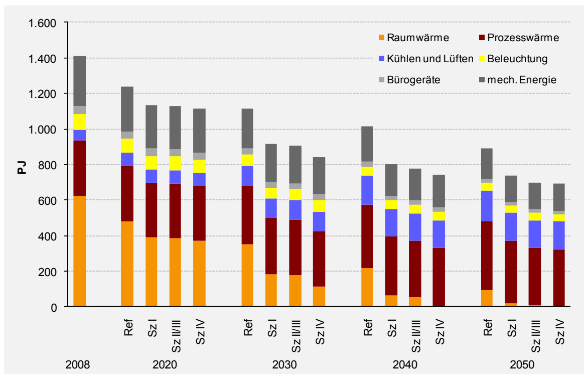
Abbildung 3.1.4-1: Endenergieverbrauch des Sektors GHD nach Verwendungszwecken 2008 – 2050 (Modellerggebnisse), in PJ
