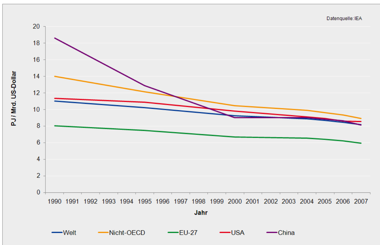
Abbildung A 2.1.1-3: Spezifischer Primärenergieverbrauch nach Regionen 1990 bis 2007, in PJ pro Mrd US-Dollar
